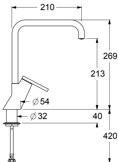
FORO UTILE HOLE WIDTH Ø35
