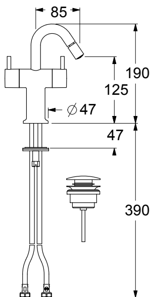
FORO UTILE HOLE WIDTH Ø35
